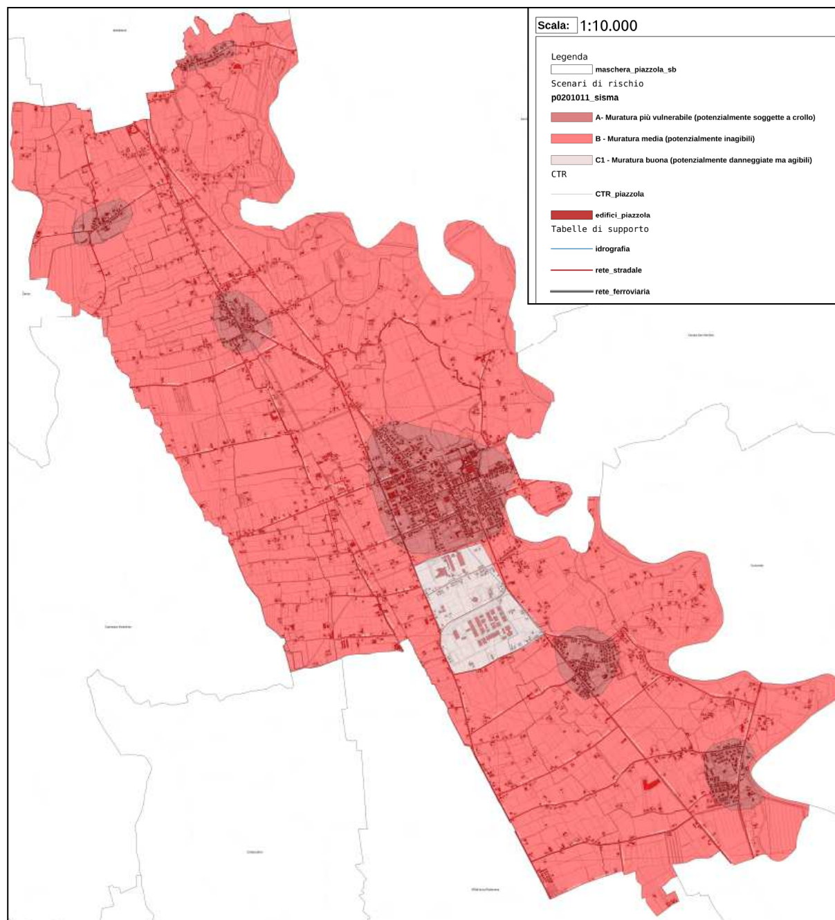
Fig. 14: diffusione della tipologia strutturale e costruttiva più comune
