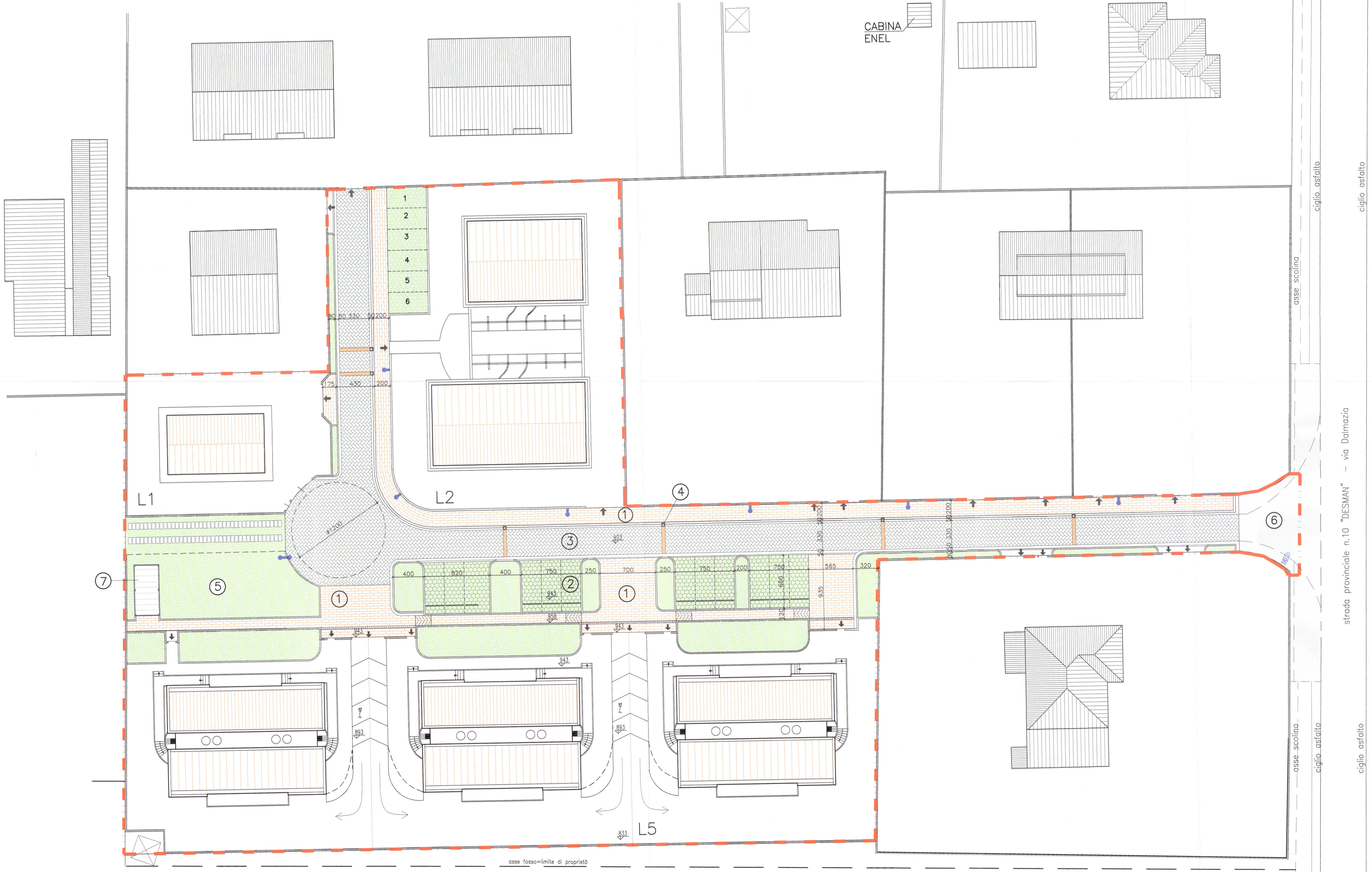
PLANIMETRIA SCALA 1:200
